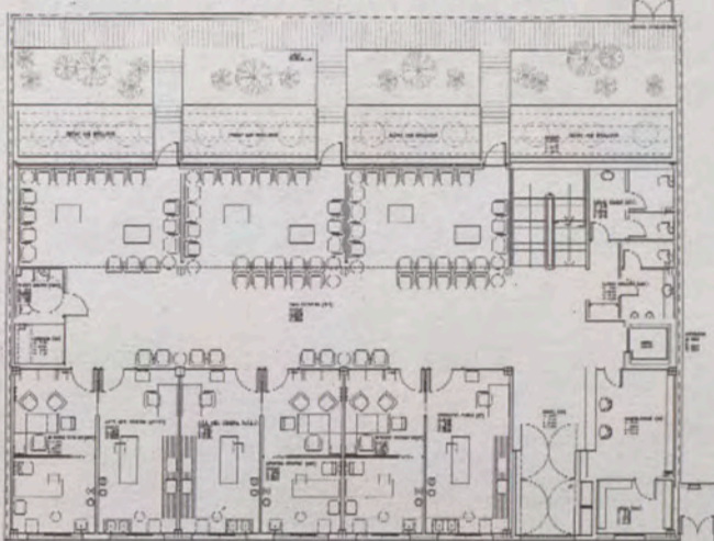
Distribució de la planta baixa de la nova unitat.
